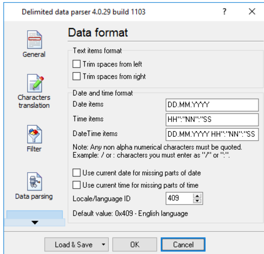
Fig. 3. Data format
