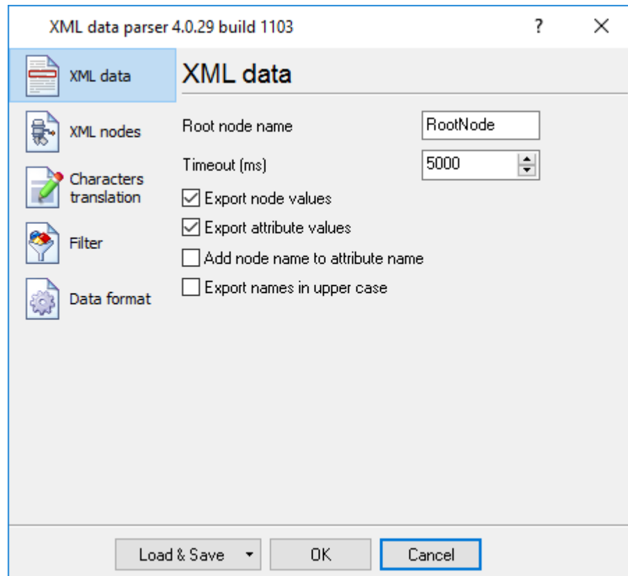
Fig.1. XML data.
