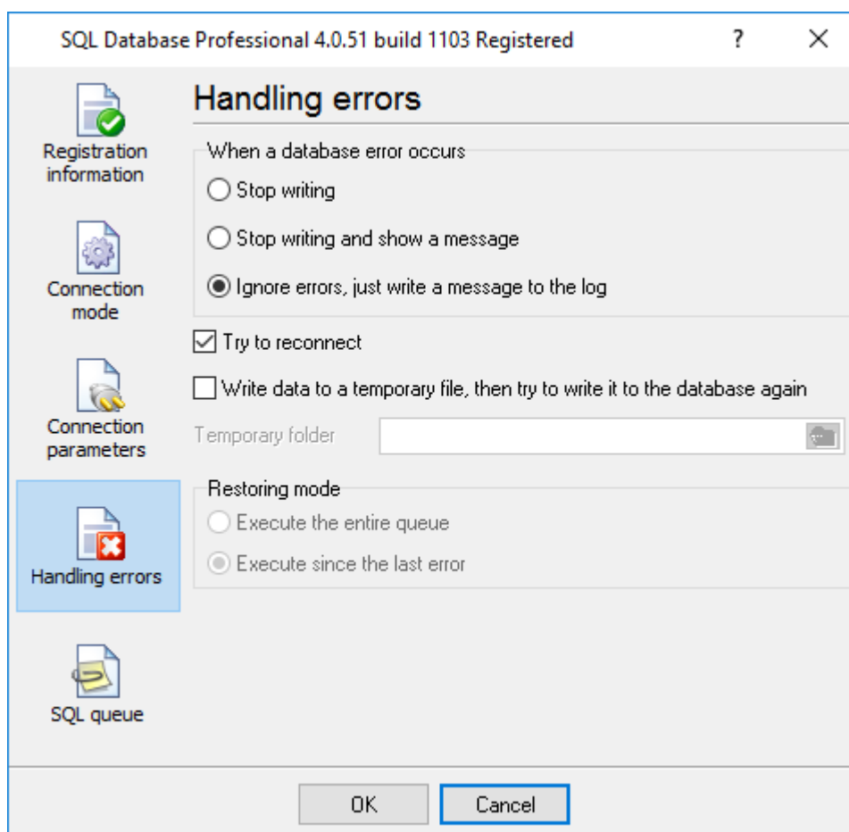
Fig. 3. Handling errors
